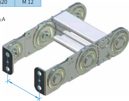
接头B
