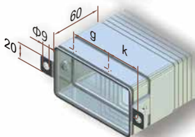
法兰 B
