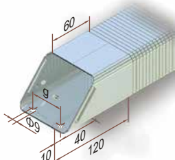
三角支架
